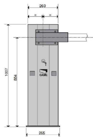
Комплект шлагбаума GARD 4000 (тумба, стрела, светоотражающие наклейки, наклейки на стрелу)
